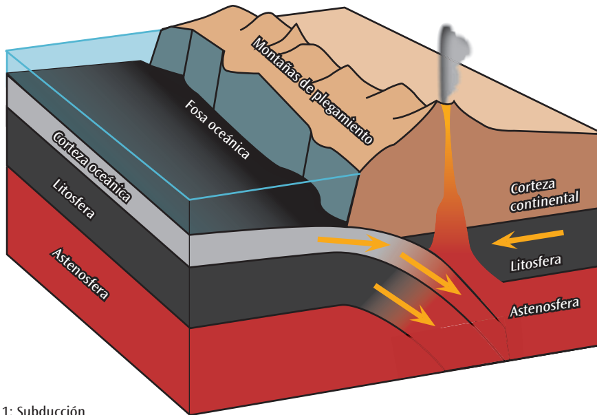
Ilustración 1: Subducción
